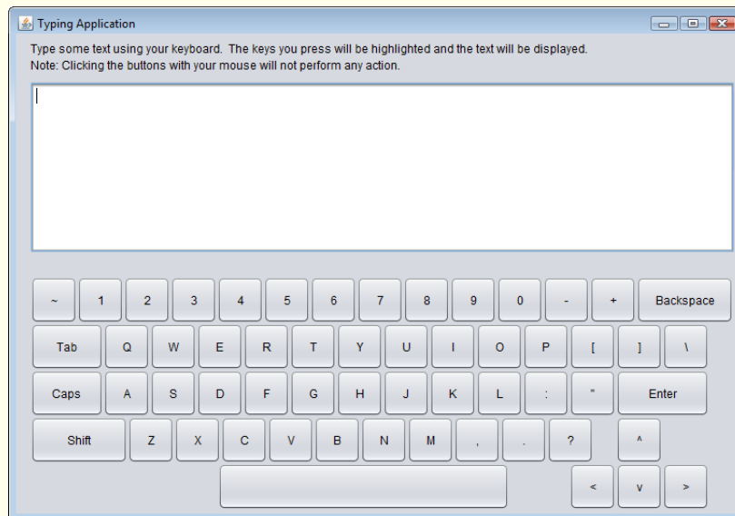
Fig. 26.50 | Typing tutor.
